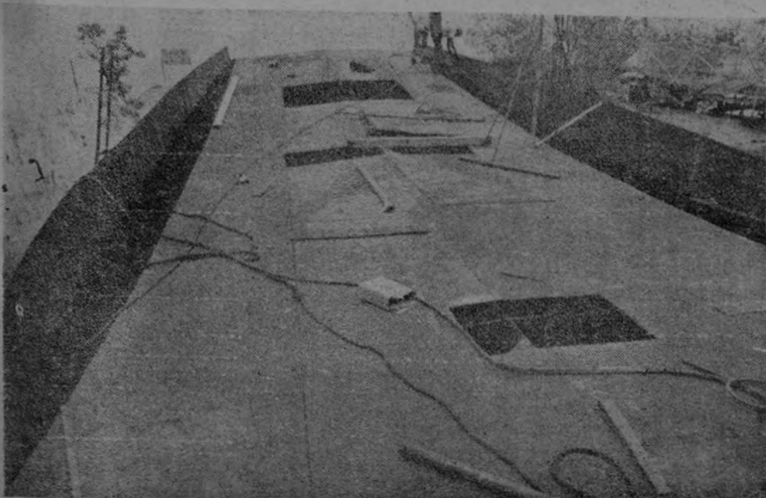
Este barco construido por astilleros nacionales está totalmente forrado en acero y con la cubierta principal ya colocada y será entregado a su propietario Sr. Rodrigo Calvo Astúa en el mes de diciembre. (Foto Córdoba).
