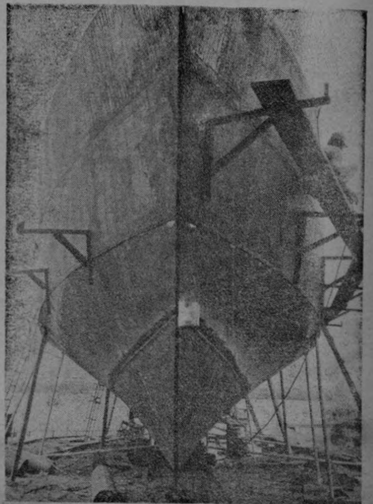
Trabajadores costarricenses realizan la construcción de un barco totalmente de acero en El Cocal de Puntarenas, como se aprecia en la gráfica. Sin embargo serán comprados dos barcos a países extranjeros, pudiendo hacerlo aquí. (Foto Córdoba).
